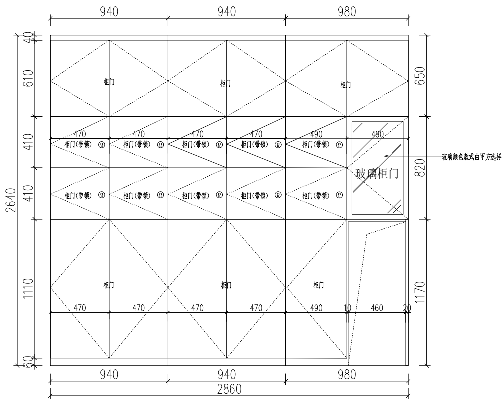
诊室定制分体造型储物柜正立面柜体
