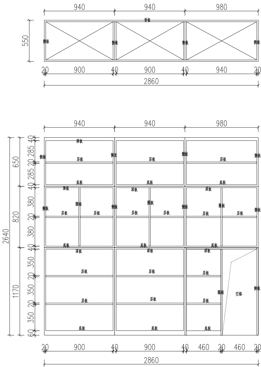
诊室定制分体造型储物柜正立面柜体
